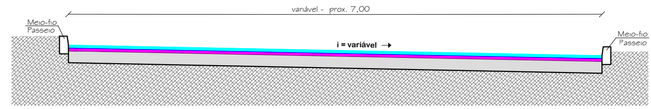
Seção Transversal B B' e espessura das camadas Av. Eliseu Rech *sem escala
