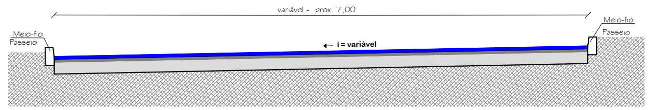
Seção Transversal A A' e espessura das camadas Av. Eliseu Rech *sem escala
