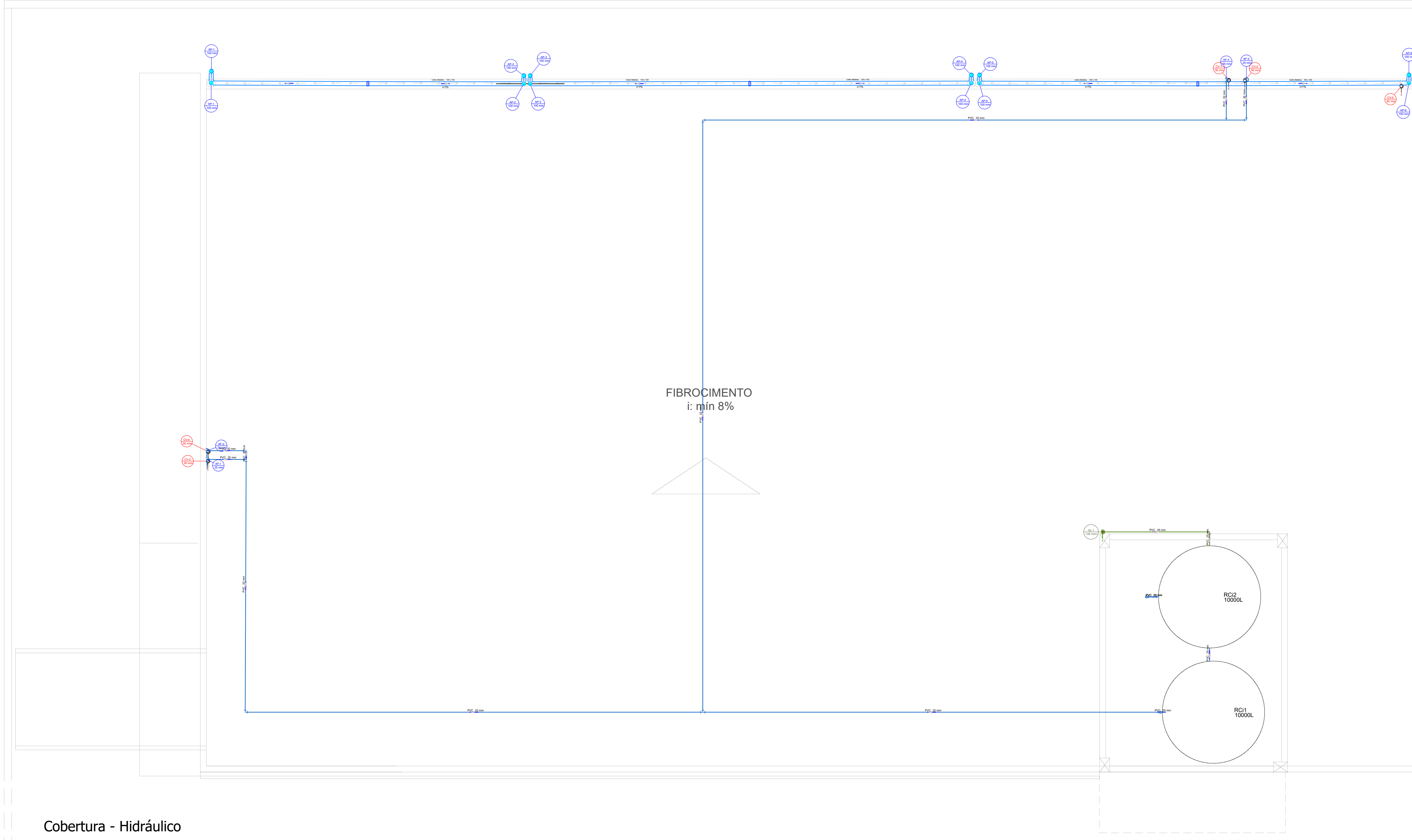
Cobertura - Hidráulico
