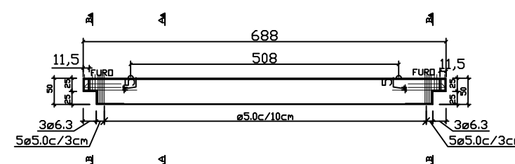
VISTA LATERAL
