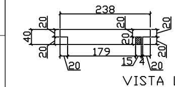
VISTA CIMA
