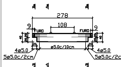
VISTA LATERAL
