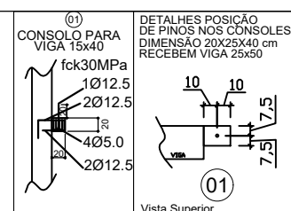
Vista Superior
