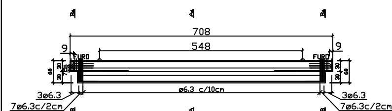
VISTA LATERAL
