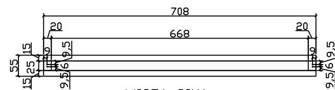
VISTA CIMA
