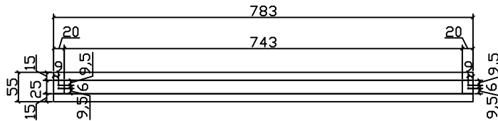
VISTA CIMA
