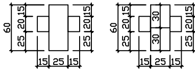
PERFIL VIGA
