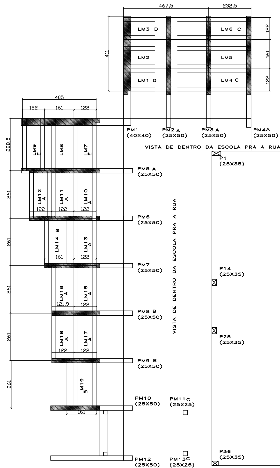
Locação Lajes Muro Contenção
