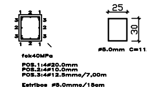
DETALHE PILAR
