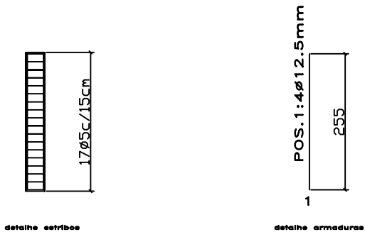
DETALHE PILAR
