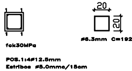
DETALHE PILAR
