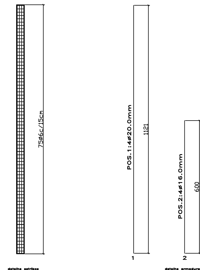
DETALHE PILAR
