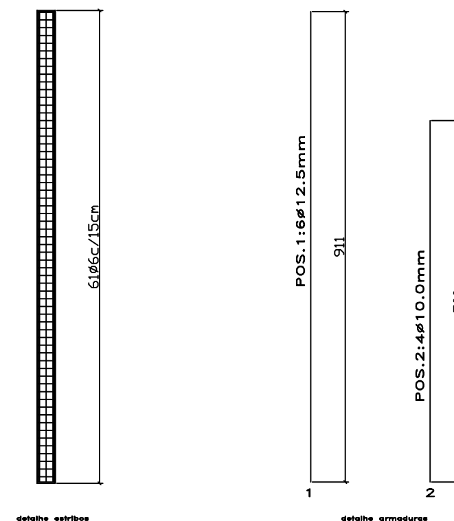
DETALHE PILAR
