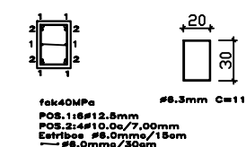
DETALHE PILAR
