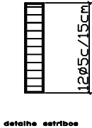
detalhe estribos
