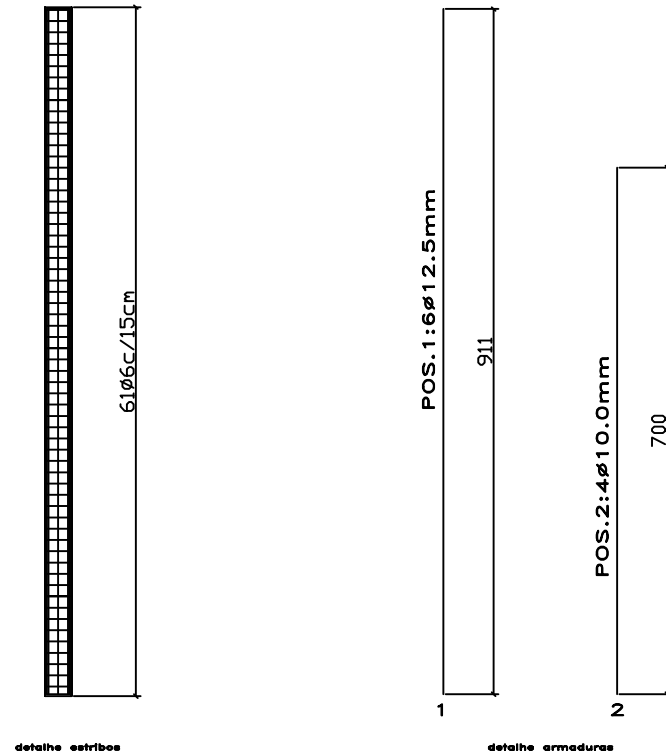
DETALHE PILAR
