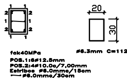
DETALHE PILAR
