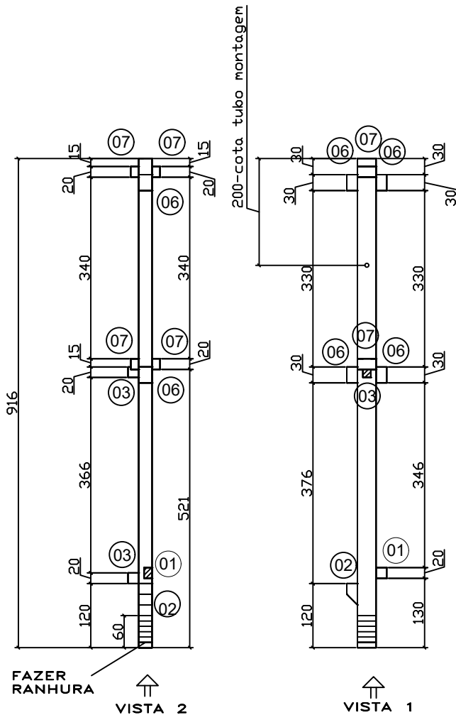
P19 (25X35)
