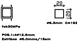
DETALHE PILAR
