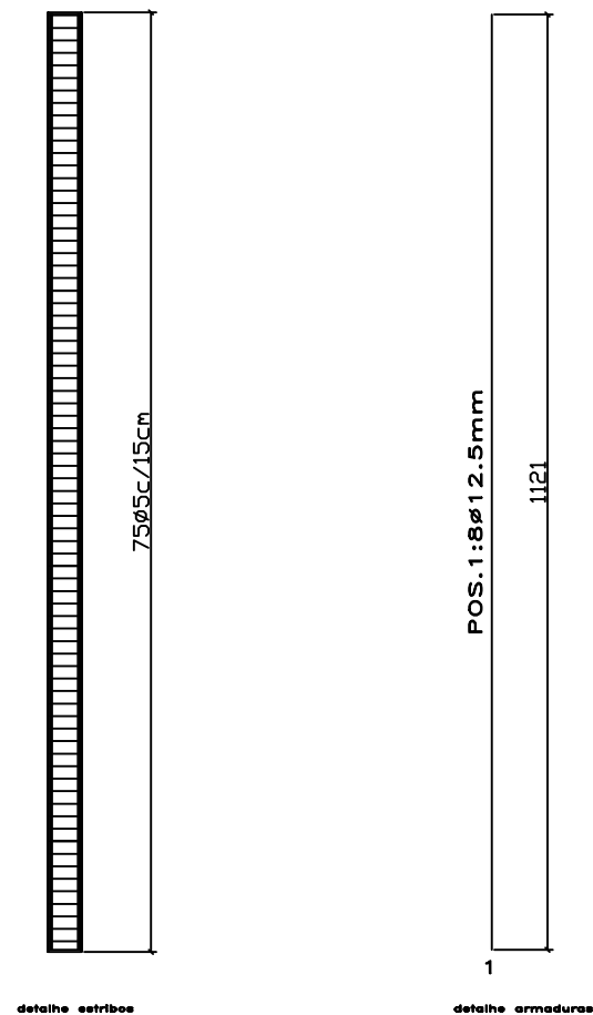
DETALHE PILAR
