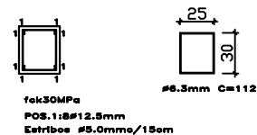
DETALHE PILAR
