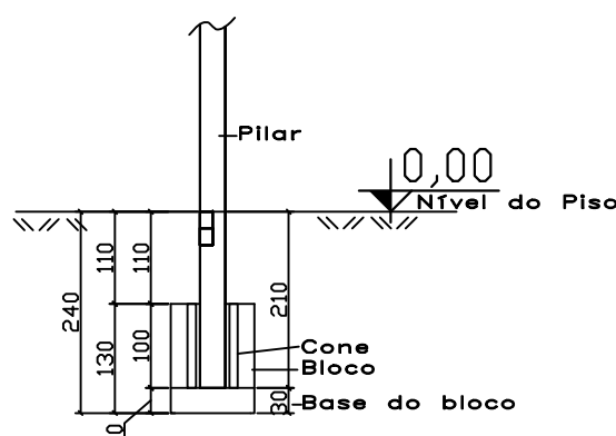
COTAS P28
