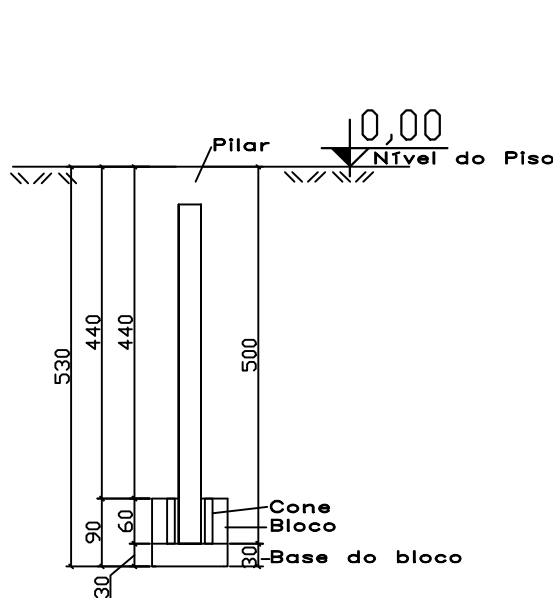
COTAS P41
