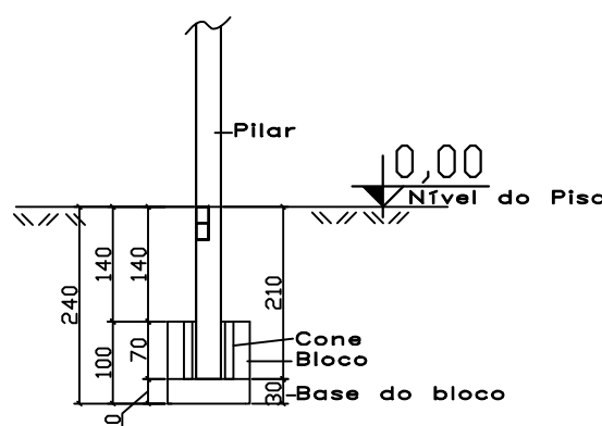
COTAS P30
