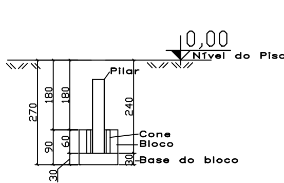
COTAS P30
