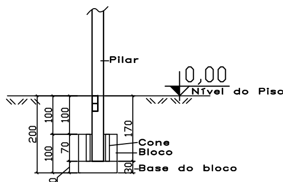
COTAS P37-P39
