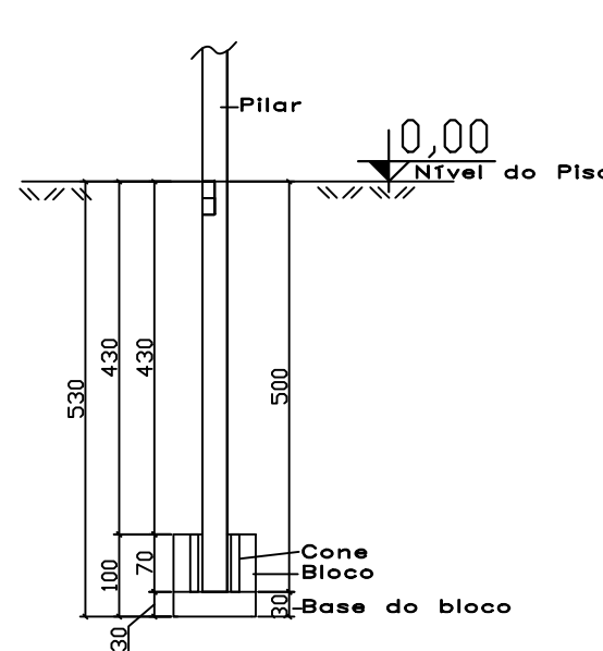
COTAS P38-P40
