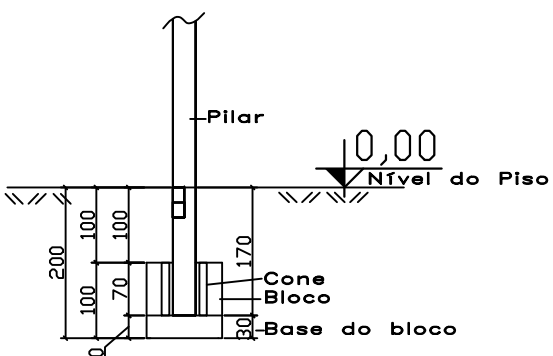
COTAS P1-P9-P23-P25-P36
