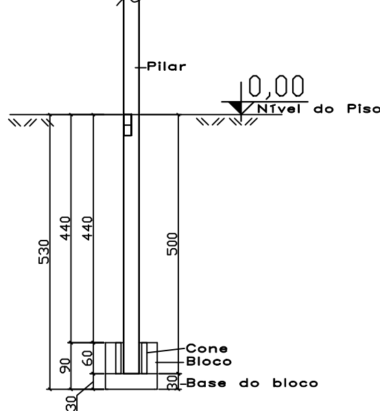
COTAS P37-P39
