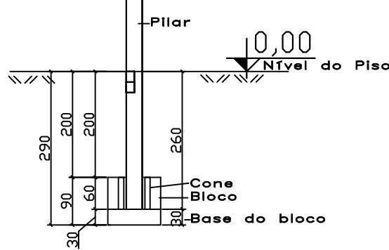
COTAS P28
