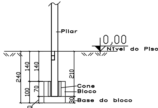
COTAS P41
