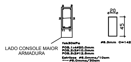
DETALHE PILAR
