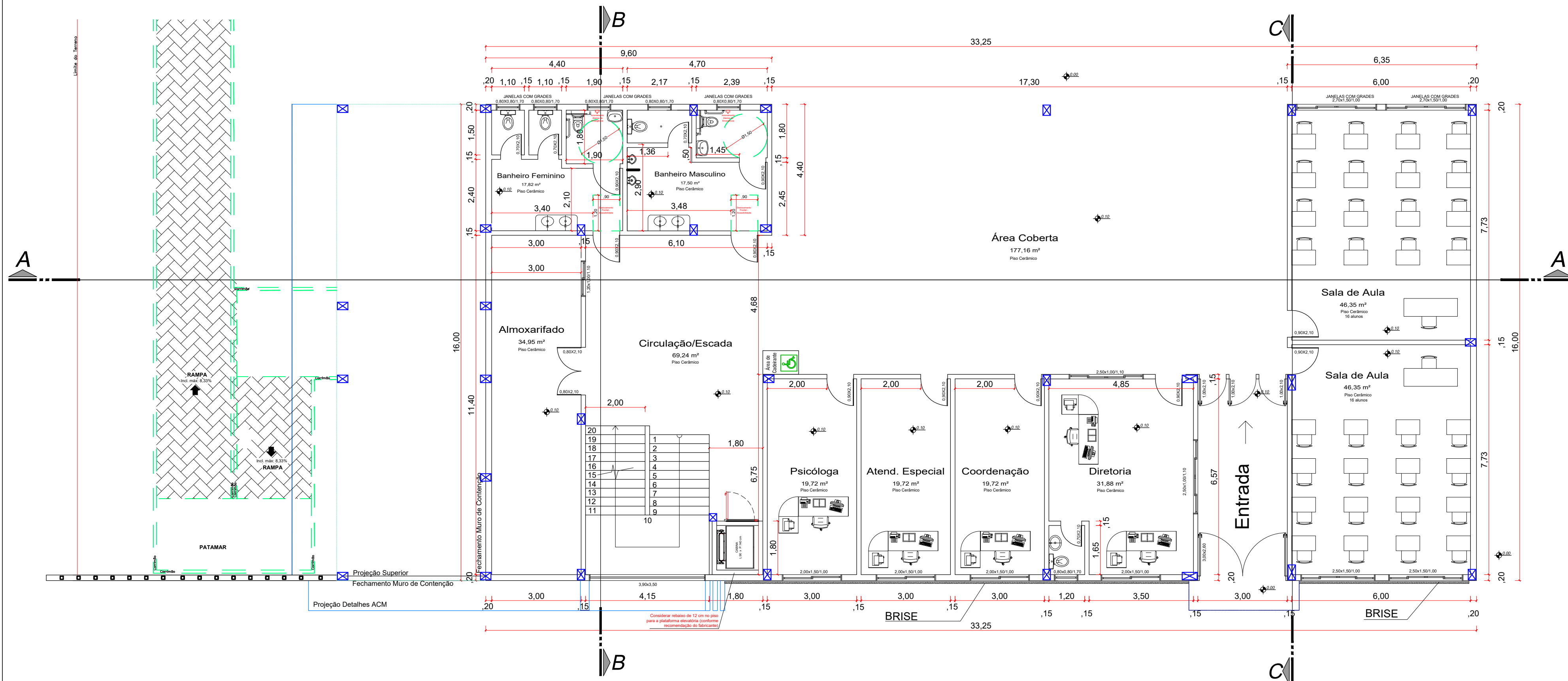
Planta Baixa Térreo 1:100 ÁREA NOVA= 532,00 m² CONFERIR MEDIDAS NO LOCAL
