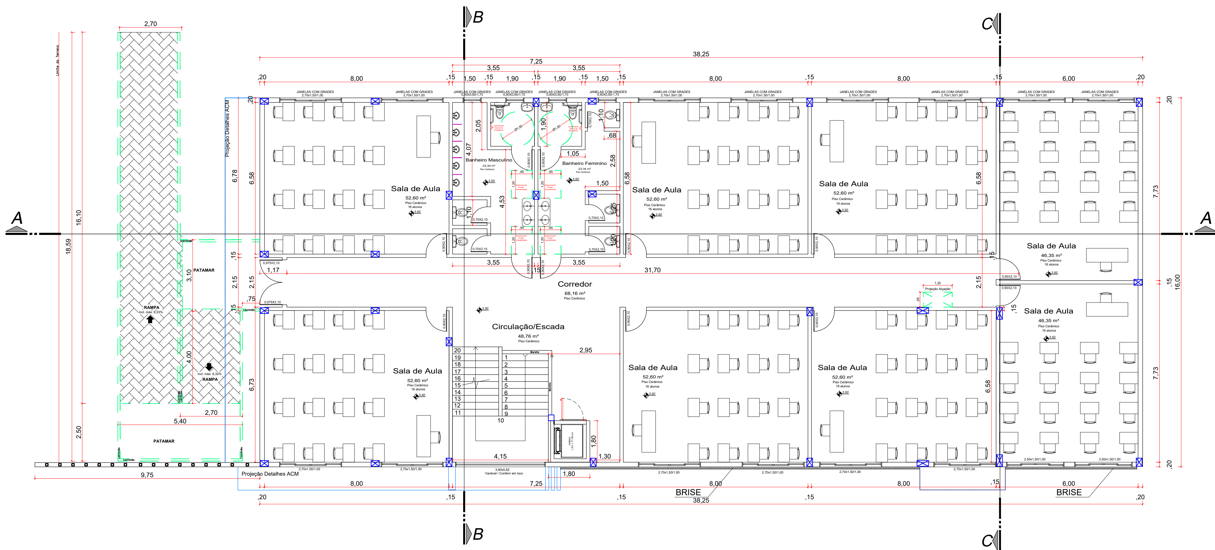
Planta Baixa Superior 1:100 ÁREA NOVA= 612,00 m² CONFERIR MEDIDAS NO LOCAL
