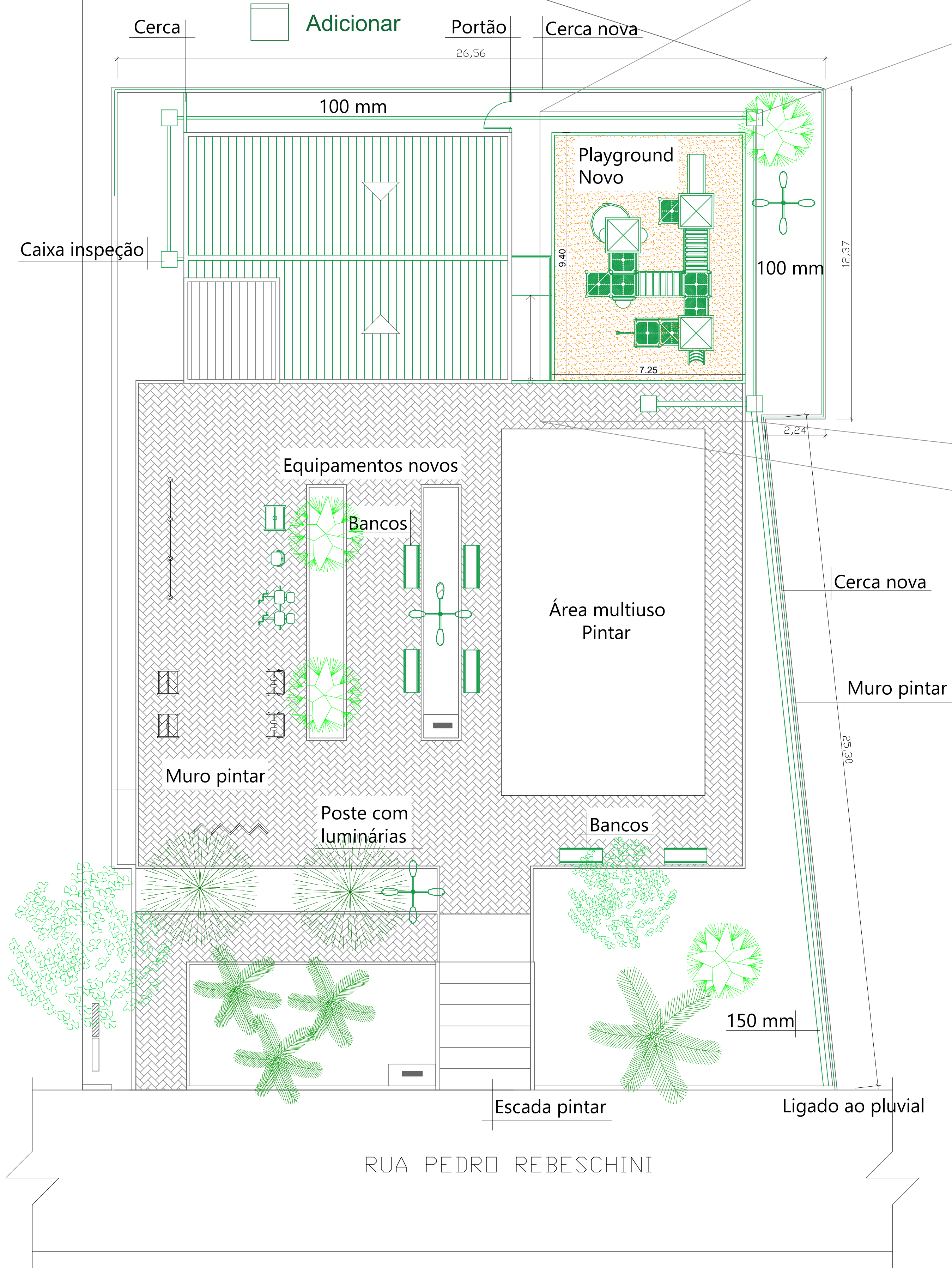
1 Implantação - Situação Final 1:100
