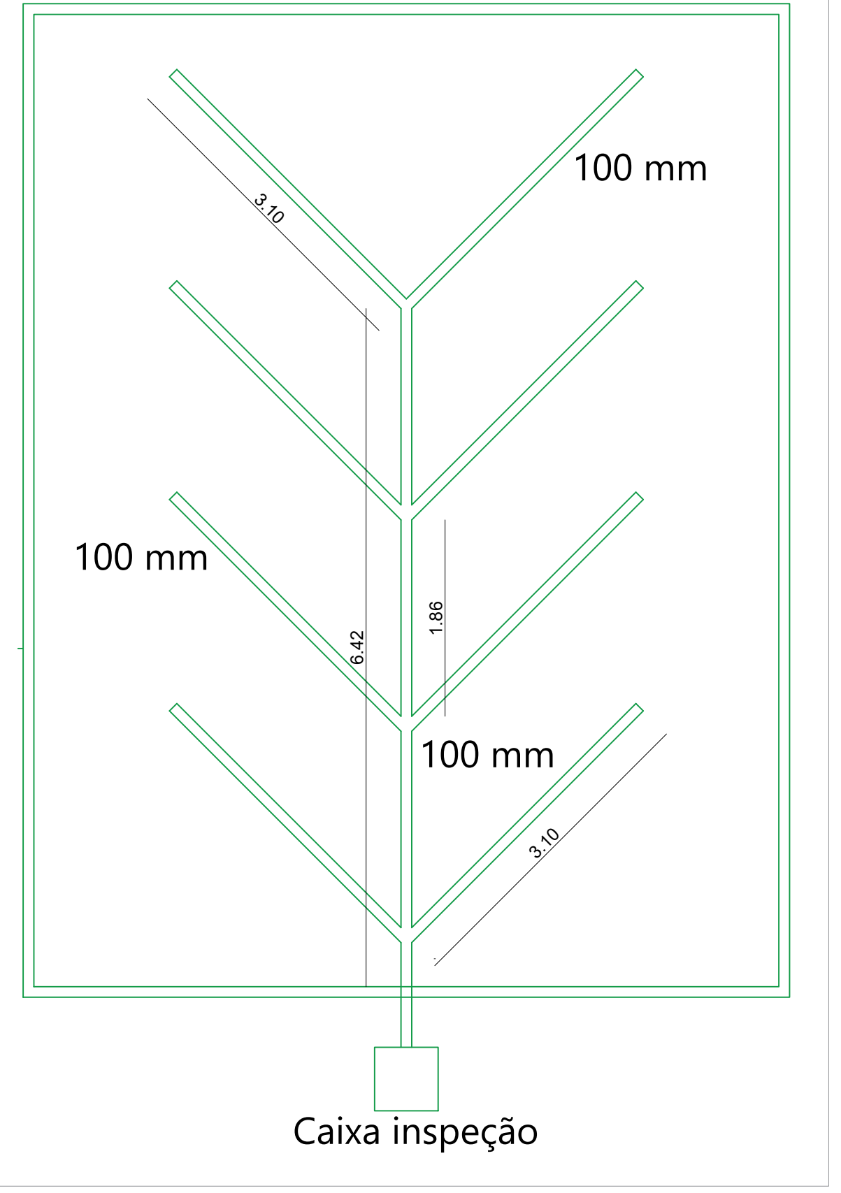
2 Detalhe Dreno Palyground 1:50
