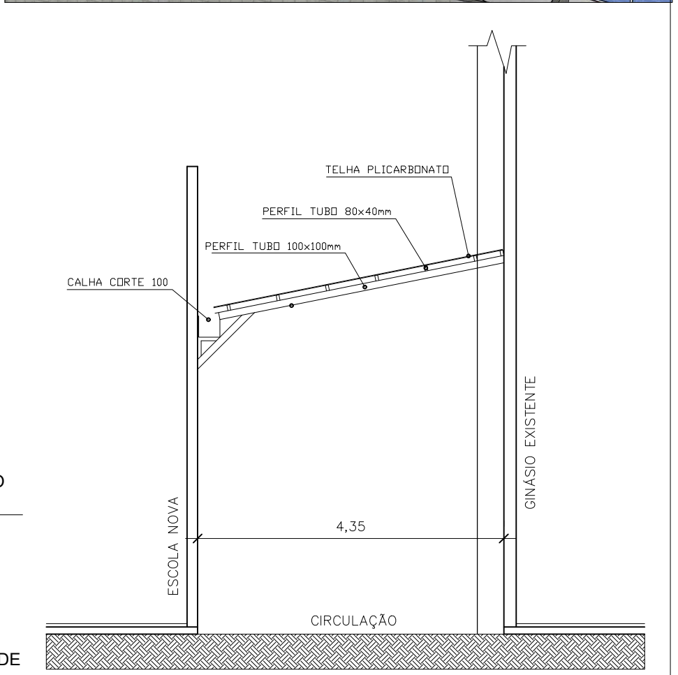
1 Corte AA' 1:75
